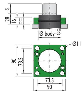
XCK-1500
