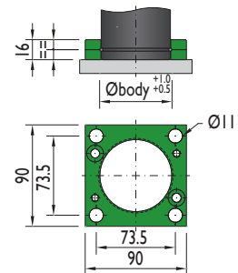
XCK-1500
